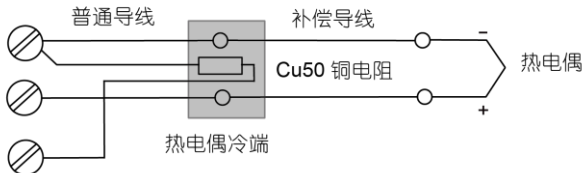
(2) 外接铜电阻自动补偿模式 (热电偶冷端接线盒最好远离发热物体)
